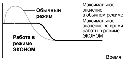
Рабочий ток и потребляемая мощность
