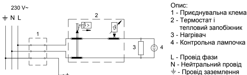
Електросхема
