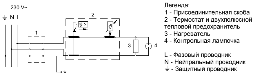
Электрическая схема
