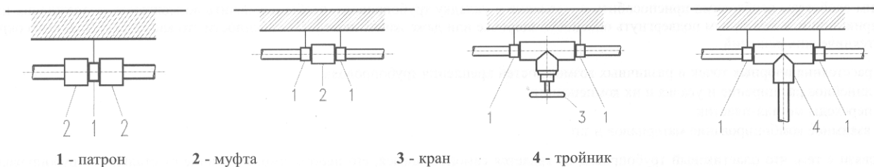
рис. 3: Примеры образования прочных опорных точек с помощью фасонины и патрона:
