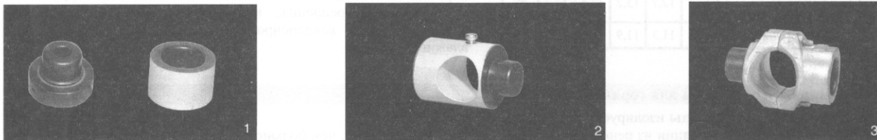
рис. 28: Полифузионные наконечники. 1) парные 2) стержневые 3) стержневые челюстные
