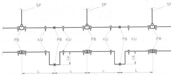
рис. 13: Классический способ компенсации горизонтального трубопровода.
