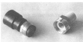
рис. 22: Пример соединения PE и PPR с помощью разборного соединения.
